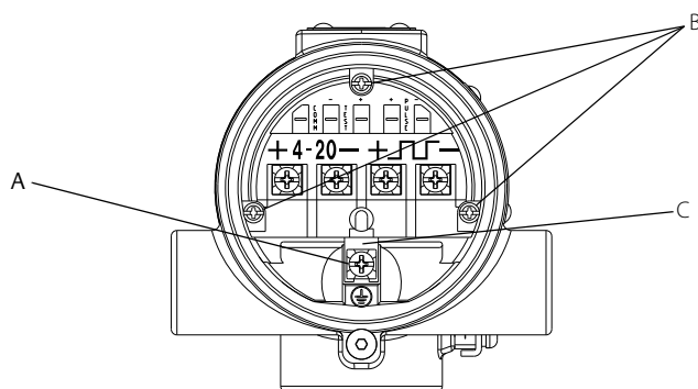
Рисунок 3-21. Клеммный блок с защитой от переходных процессов
