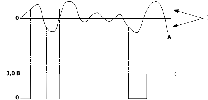
Рисунок 5-5. Неправильный размер/фильтрация
