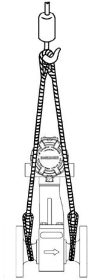
Рисунок 3-7. Универсальный строп
