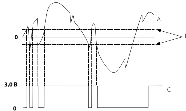
Рисунок 5-4. Искаженные сигналы
