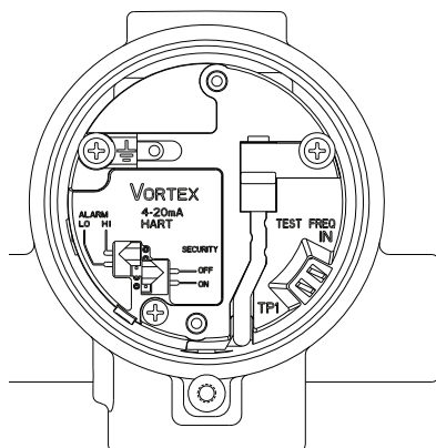
Рисунок 3-5. Переключки аварийной сигнализации и защиты
